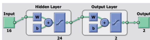
شکل ۳. لایه‌ها و تعداد نرون‌های شبکه طراحی شده
